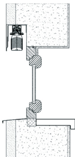
Montaż żaluzji w nadprożu
