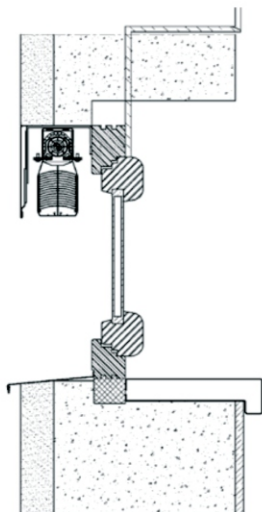
Montaż żaluzji na ramie okna
