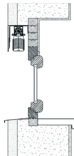
Montaż żaluzji do poszerzenia
